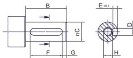
Конец вала, шпоночный паз (опция)
