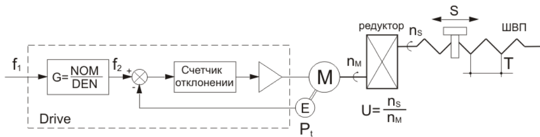
Рисунок 6-6 Функциональная схема электропривода для определения электрического шага G
