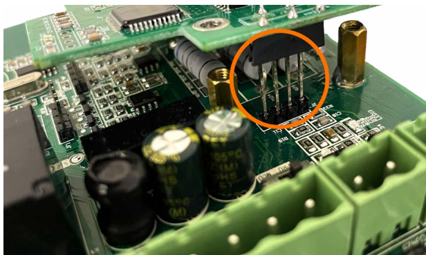
Рисунок 18 – Установка платы расширения SNI-DP-B к плате управления SNI
