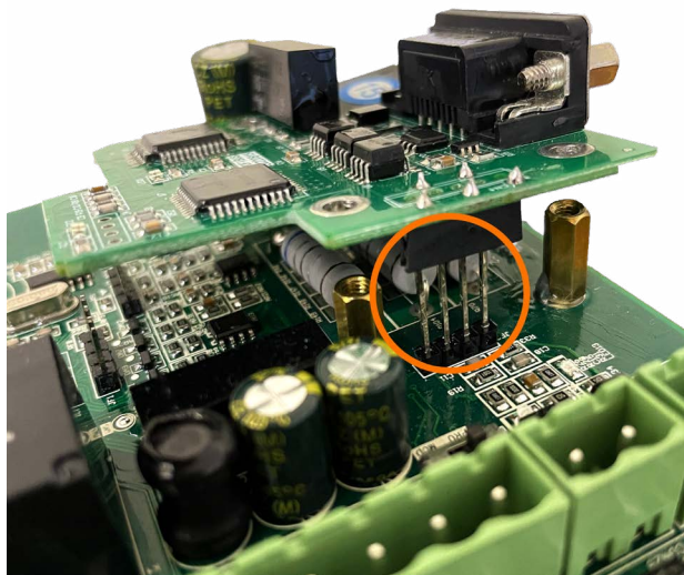
Рисунок 9 – Установка платы расширения SNI-DP-S к плате управления SNI
