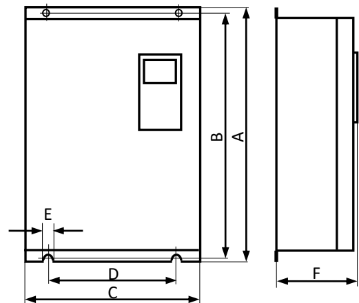
Рисунок 2 18,5...160 кВт (025Н...200Н)
