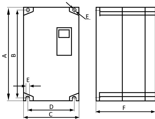
Рисунок 1 1,5...15 кВт (002Н...020Н)
