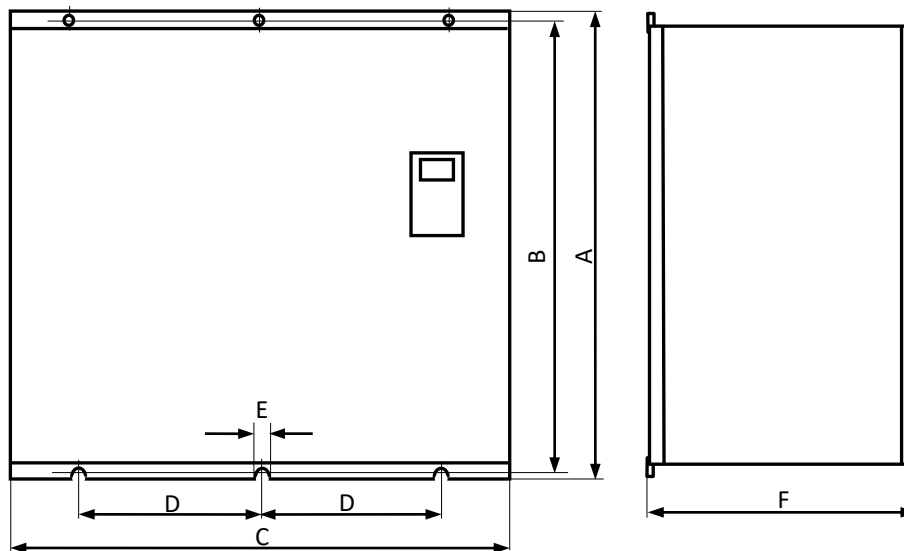
Рисунок 3 220...315 кВт (300Н...400Н)
